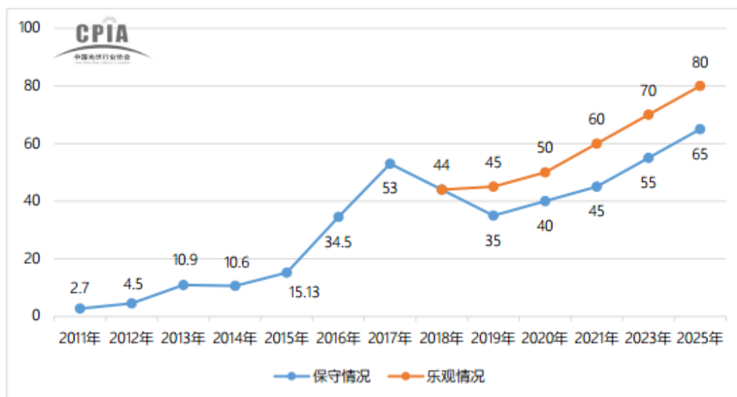
2011-2018 年国内光伏年度新增装机规模以及 2019-2025 年新增规模预测（单位：GW）
