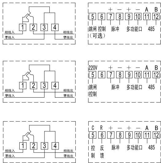
图 3：直接接入式
