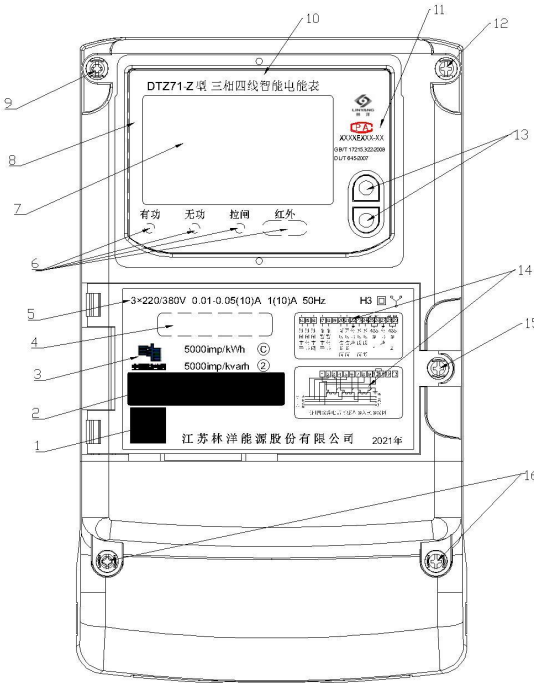
图2 外形图
