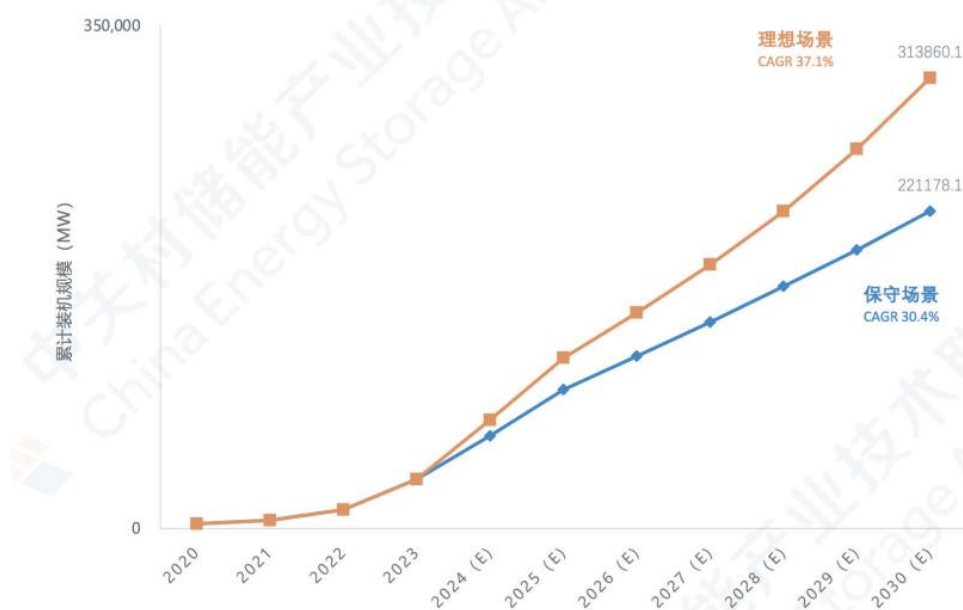
图 1：中国新型储能累计投运装机规模预测（2024-2030 年）（单位：MW）
